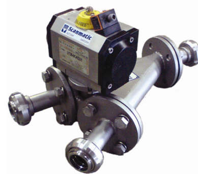
Växventil utrustat med manöverdon och gränsläge.
